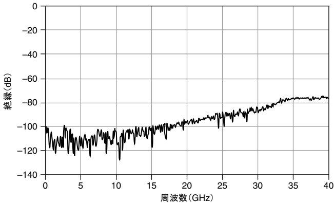
図 2. 標準絶縁
