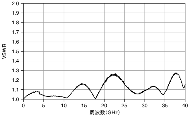
図 3. 標準 VSWR
