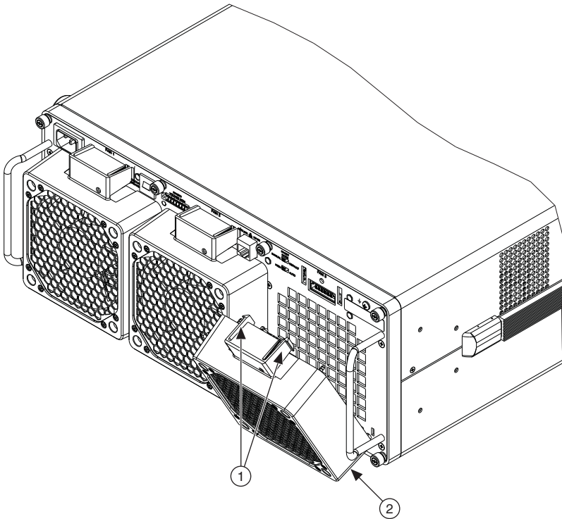
Figure 1. Replacing Fan Module
